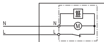
Схема соединений
