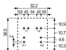
Вид сбоку
